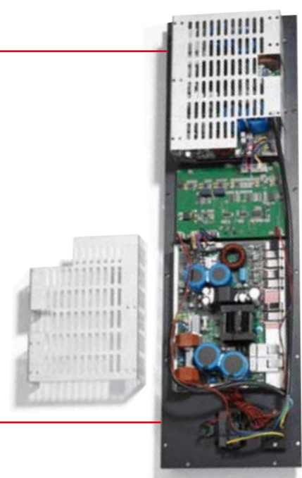
Links und rechts gegensätzlich montierte Tieftöner lassen dem Anwender die Wahl nach innen oder außen gerichteter Bässe. Die komplexe Elektronik (oben) ist im hinteren Teil der Box untergebracht.
